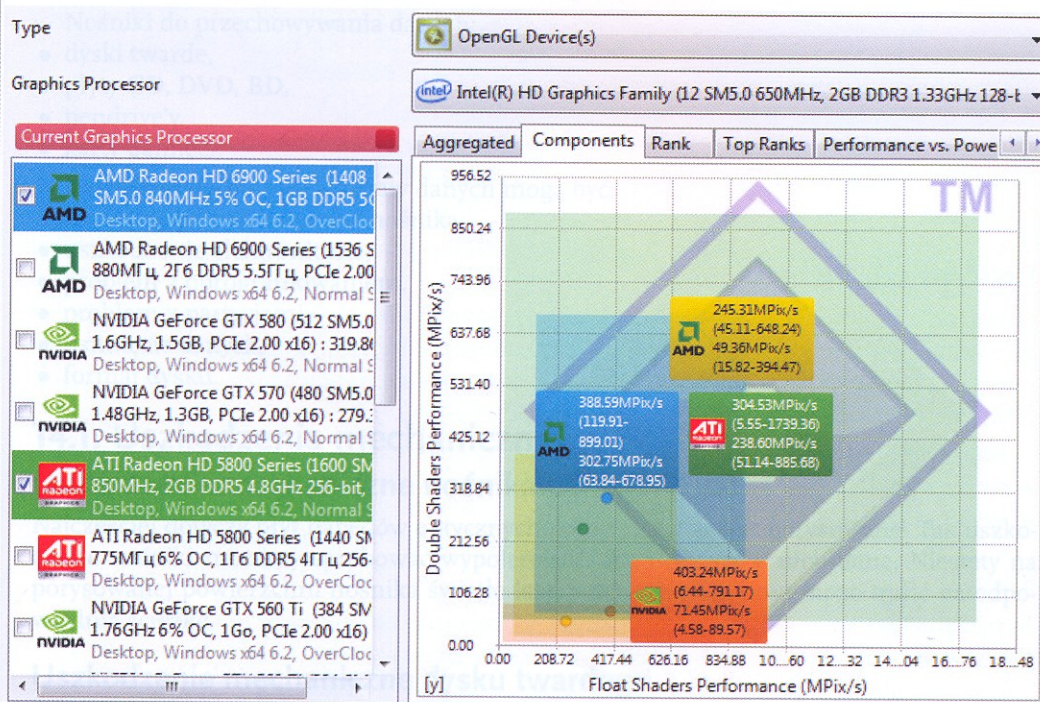
Rys. 13.13. Moduł Video Rendering w programie Sisoft Sandra
