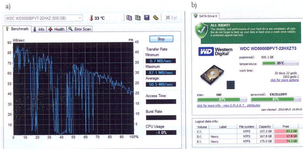
Rys. 13.11. a) Wyniki testu HD Tune, b) Monitor dysku programu HDDlife
