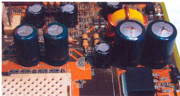
Rys. 3.2. Przykład dobrych kondensatorów (po lewej) oraz napuchniętych (po prawej)
